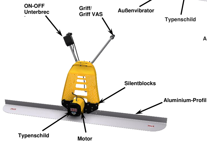
VIBRIERPATSCH MIT ELEKTRISCHEM ODER BENZINMOTOR "TORNADO"
