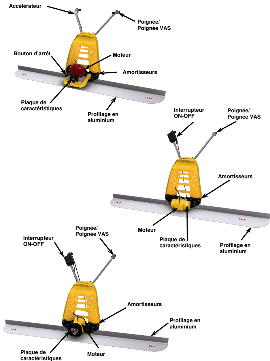
RÈGLES VIBRO-LISSEUSES À MOTEUR ÉLECTRIQUE OU ESSENCE "TORNADO"
